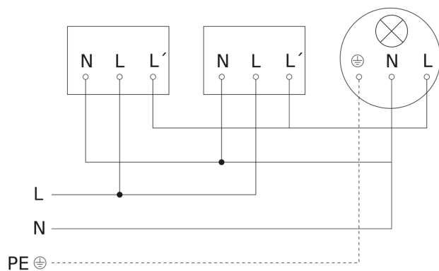
Diagrama electrónico interconexión varios sensores
