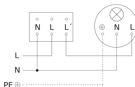
Diagrama electrónico cableado de 3 hilos
