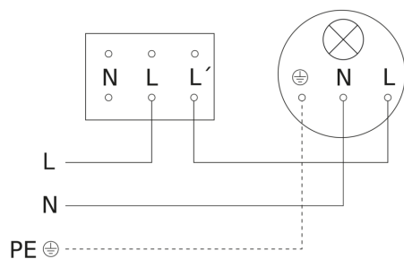
Diagrama electrónico cableado de 2 hilos
